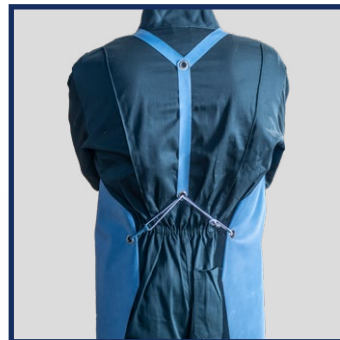
Tablier BRAVO avec montage harnais BRAVO apron with harness fitting
